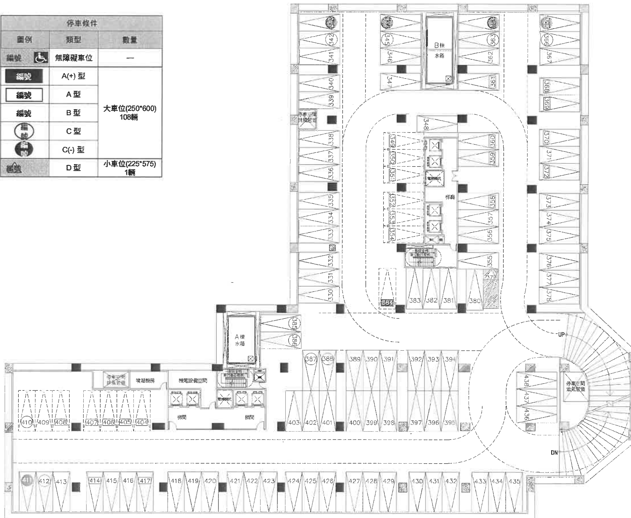
圖 13-3 地下二層更新後停車位分配單元及位置對照圖
