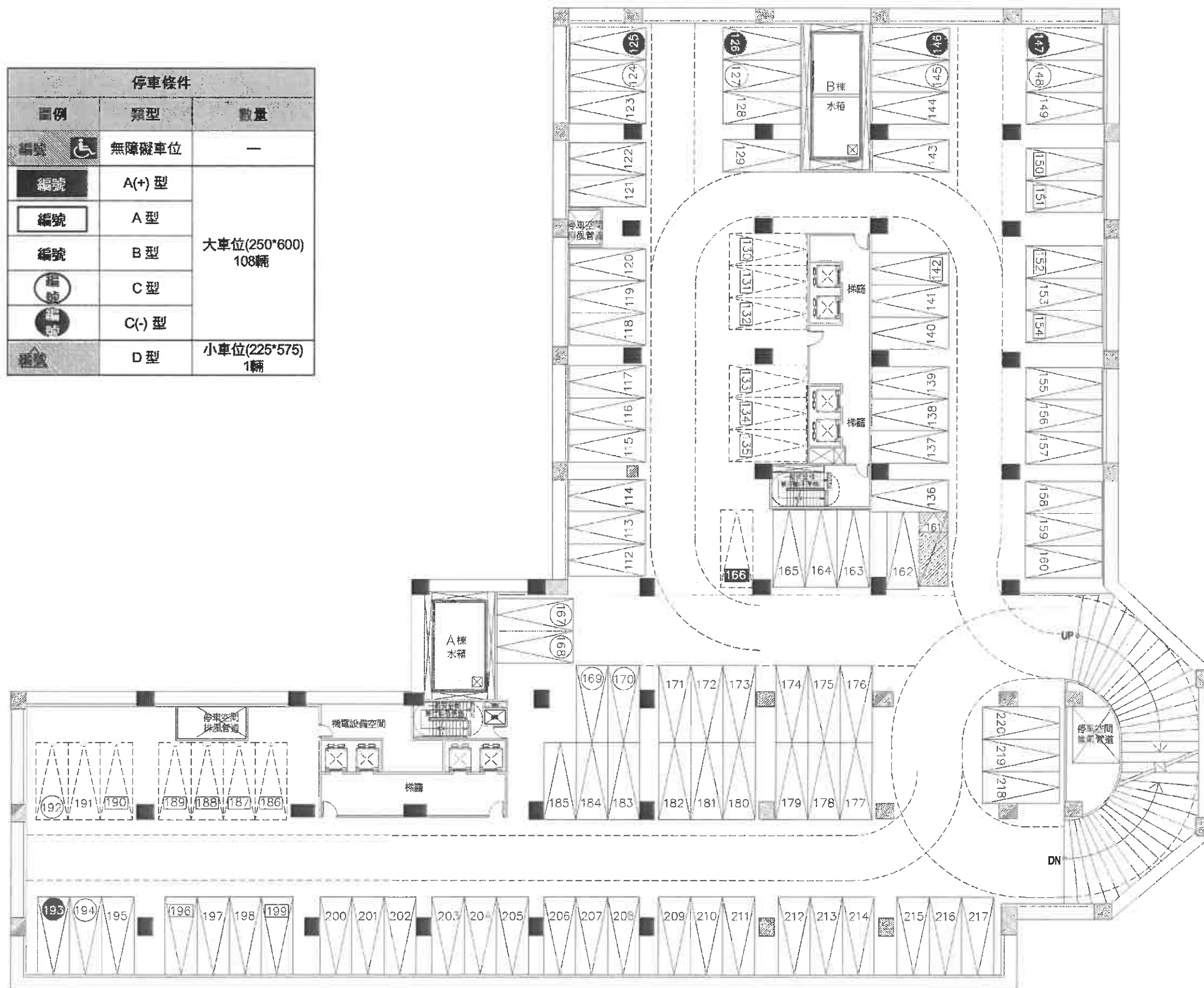
圖 13-5 地下四層更新後停車位分配單元及位置對照圖
