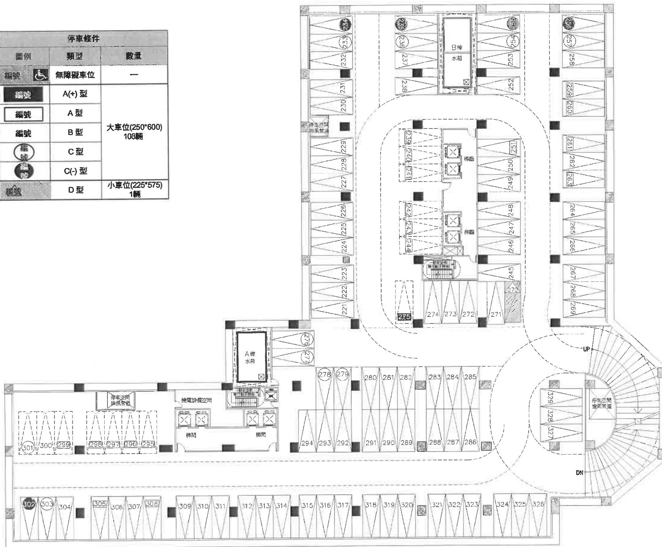
圖 13-4 地下三層更新後停車位分配單元及位置對照圖
