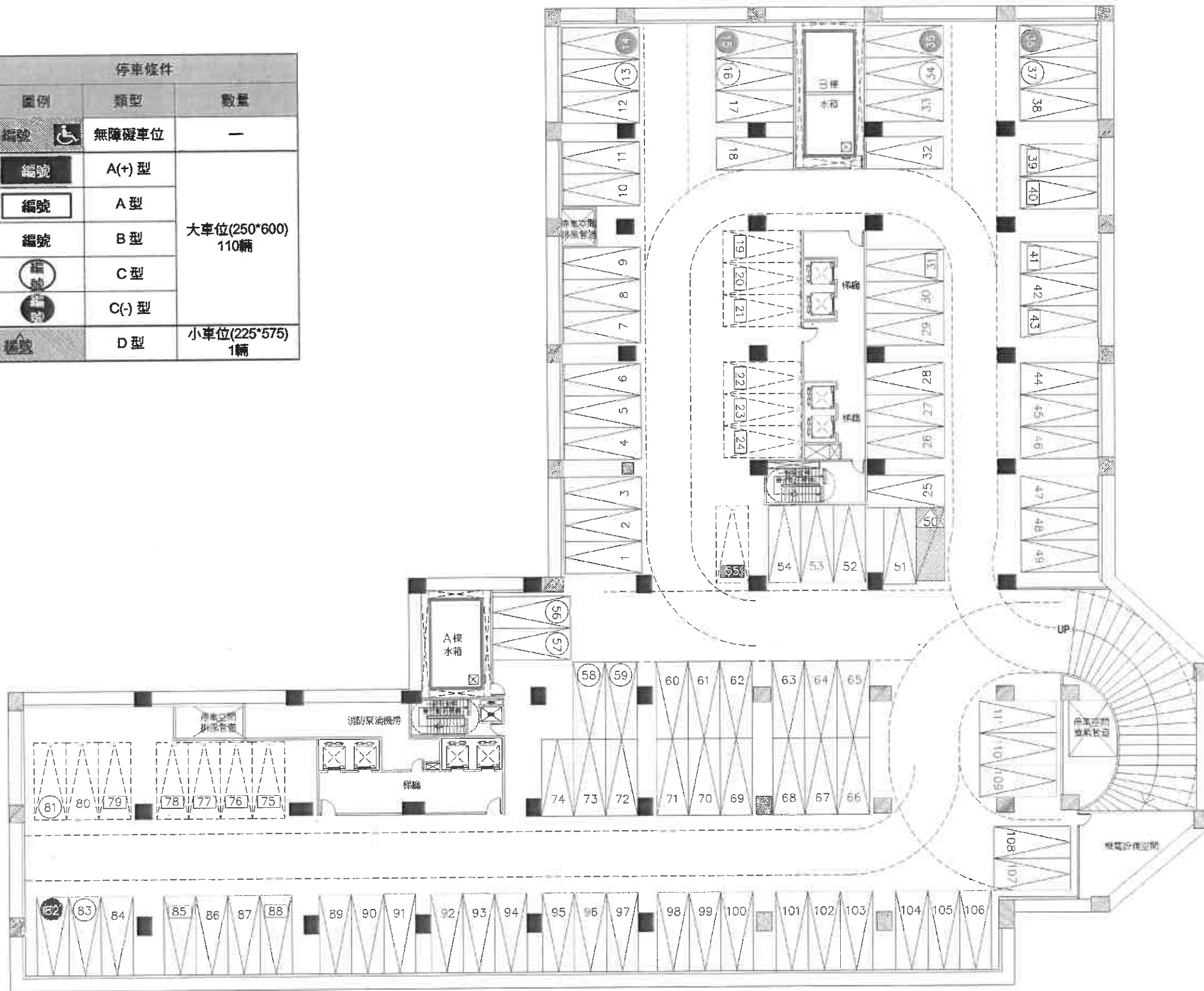
圖 13-6 地下五層更新後停車位分配單元及位置對照圖
