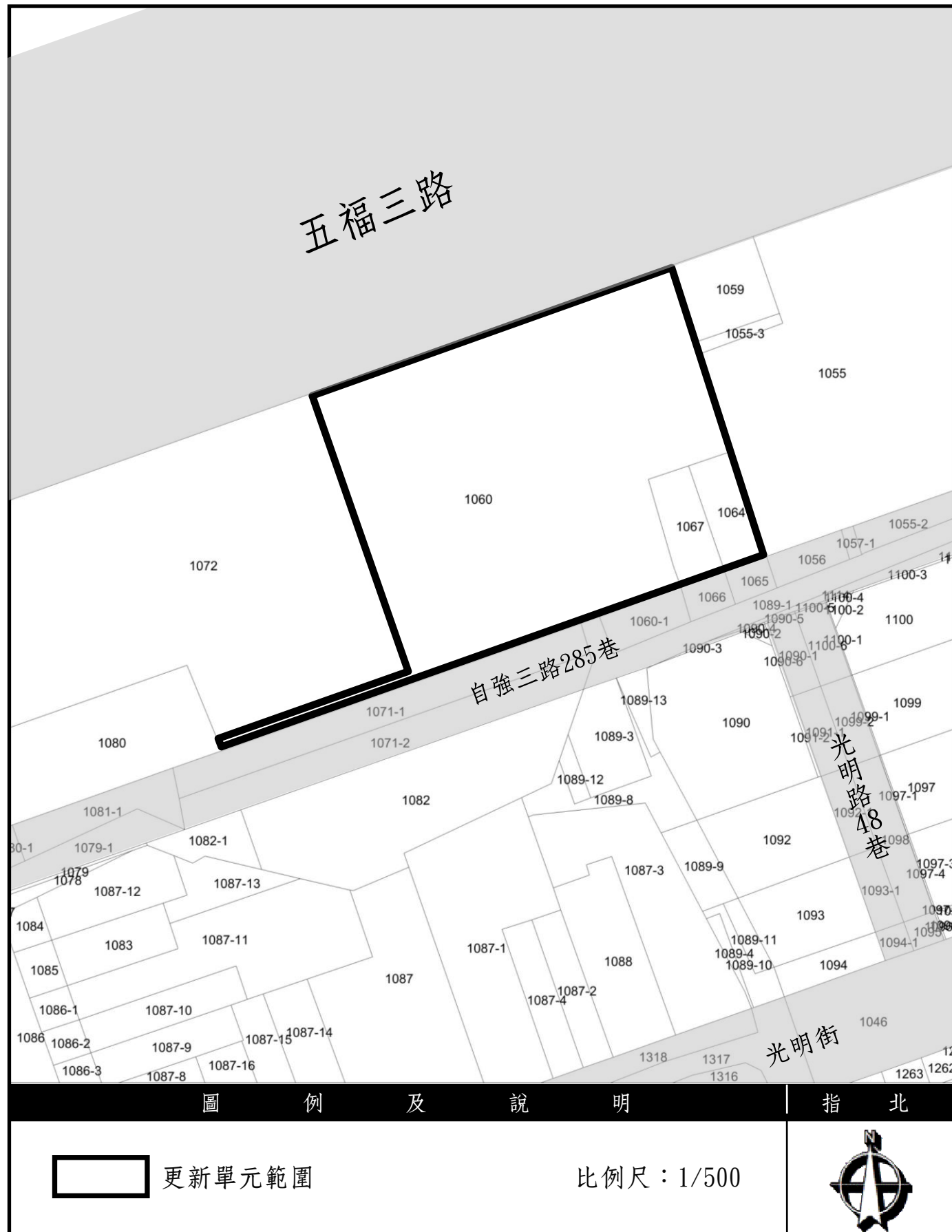
圖 2-2 權利變換地區地籍套繪圖
